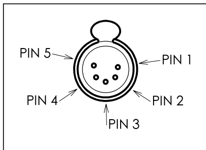
Grafik 12 - 4: DMX-Ausgang
