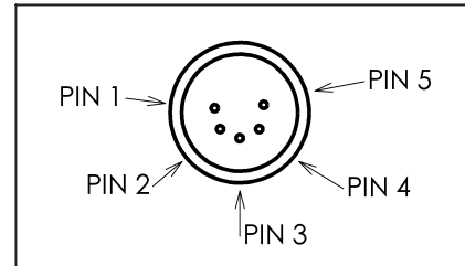
Grafik 12 - 7: DMX-Eingang
